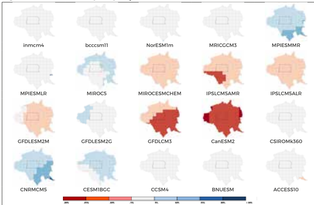
Figura 25 - Anomalia da precipitação total - RCP4.5 w/m 2 - 2011 a 2040.
