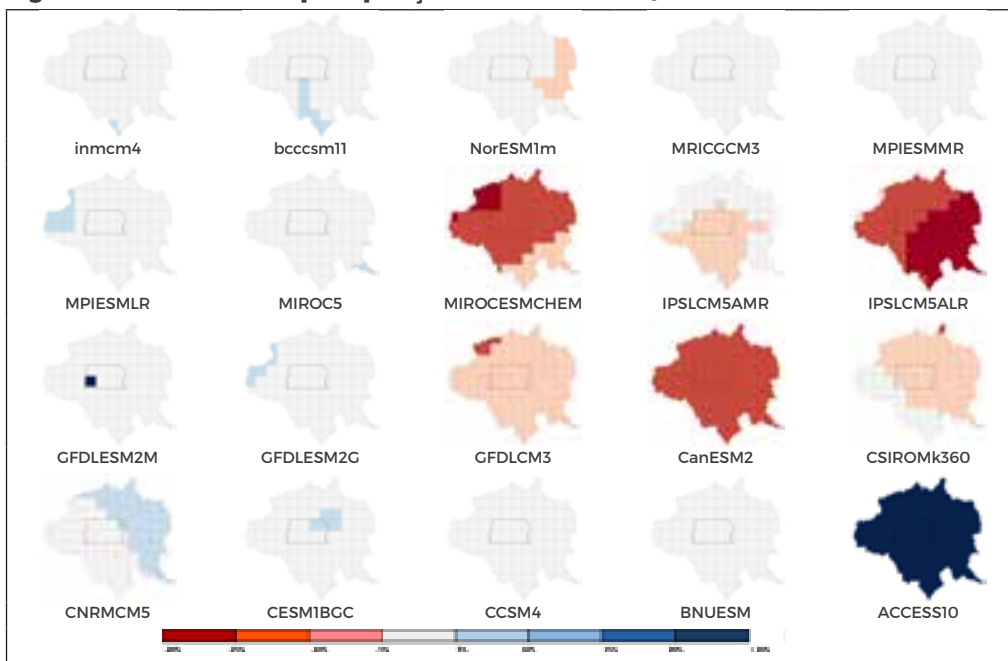
Figura 26 - Anomalia da precipitação total - RCP8.5 w/m 2 - 2011 a 2040.
