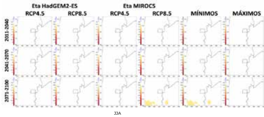
JJA
