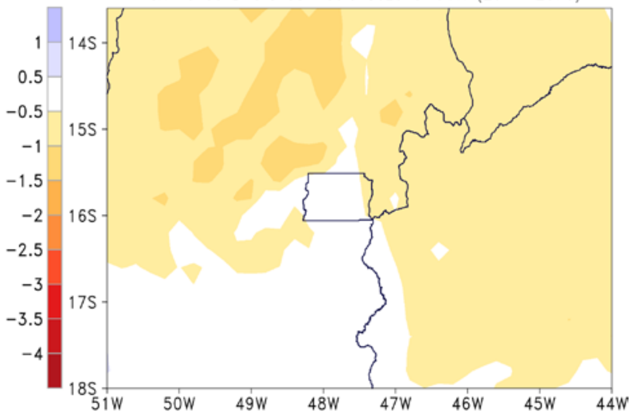
Precipitacao (mm/dia) Eta HadGEM2-ES+MIROC5 20km Maximo da Diferença Media Sazonal SON (2041-2070)
