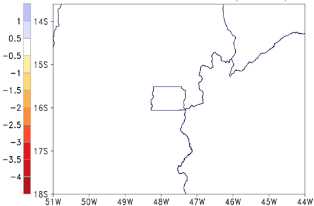
Precipitacao (mm/dia) Eta HadGEM2-ES+MIROC5 20km Minimo da Diferenca Media Sazonal JJA (2041-2070)
