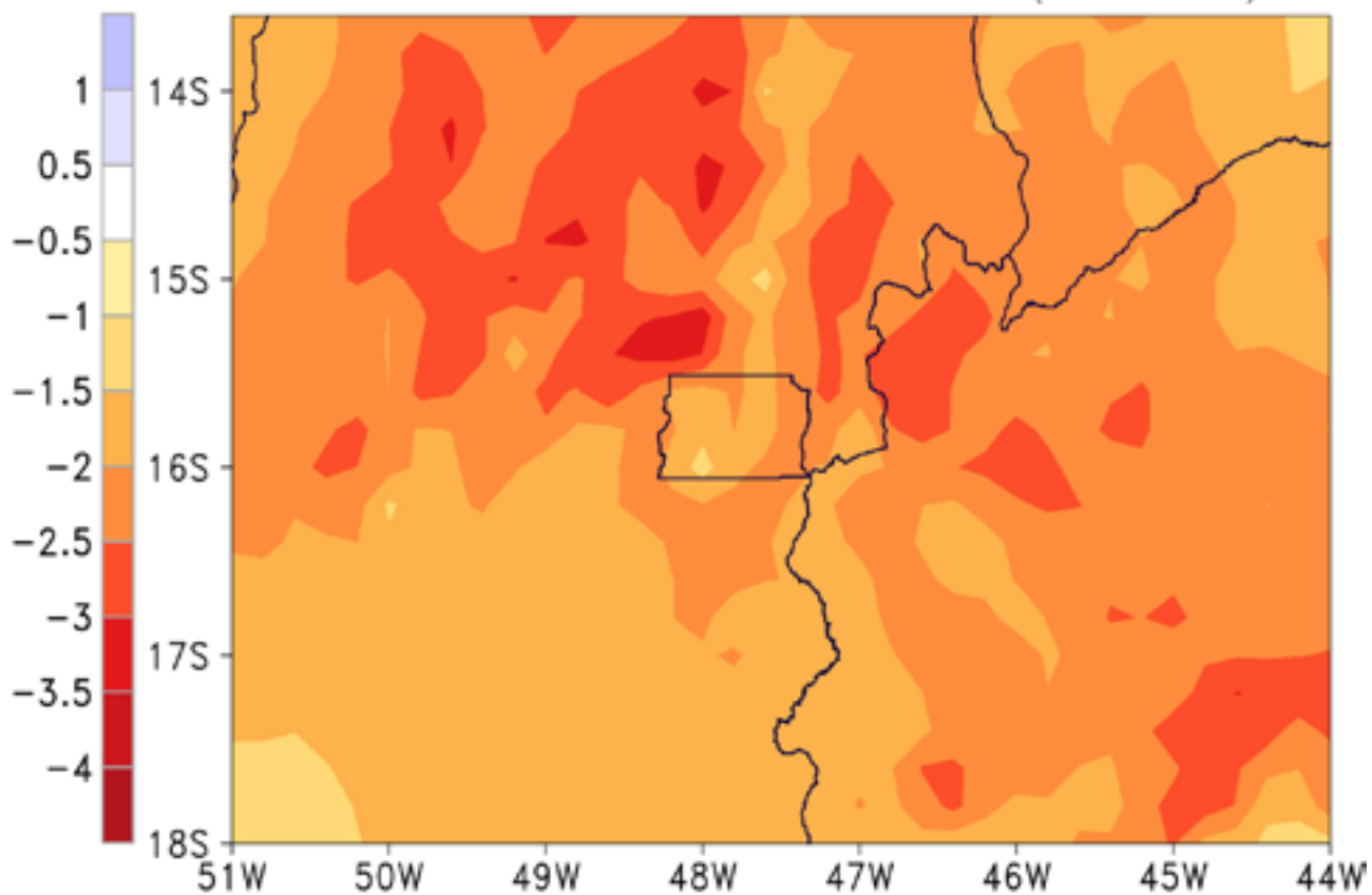
Precipitacao (mm/dia) Eta HadGEM2-ES+MIROC5 20km Mínimo da Diferença Média Sazonal SON (2071-2099)
