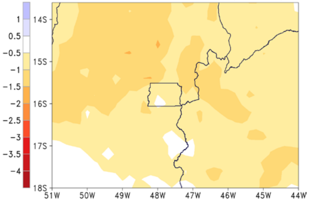
Precipitacao (mm/dia) Eta HadGEM2-ES+MIROC5 20km Maximo da Diferenca Media Sazonal SON (2011-2040)
