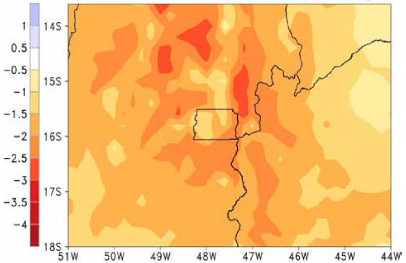
Precipitacao (mm/dia) Eta HadGEM2-ES+MIROC5 20km Mínimo da Diferença Média Sazonal MAM (2011-2040)
