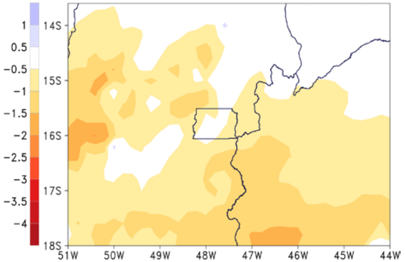
Precipitacao (mm/dia) Eta HadGEM2-ES+MIROC5 20km Maximo da Diferenca Media Sazonal DJF (2041-2070)
