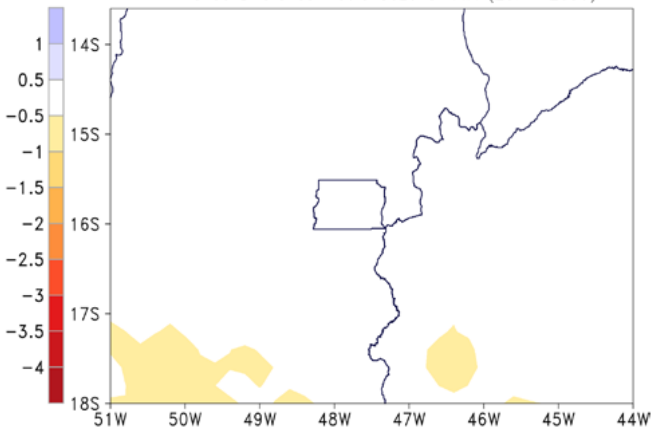
Precipitacao (mm/dia) Eta HadGEM2-ES+MIROC5 20km Minimo da Diferenca Media Sazonal JJA (2071-2099)
