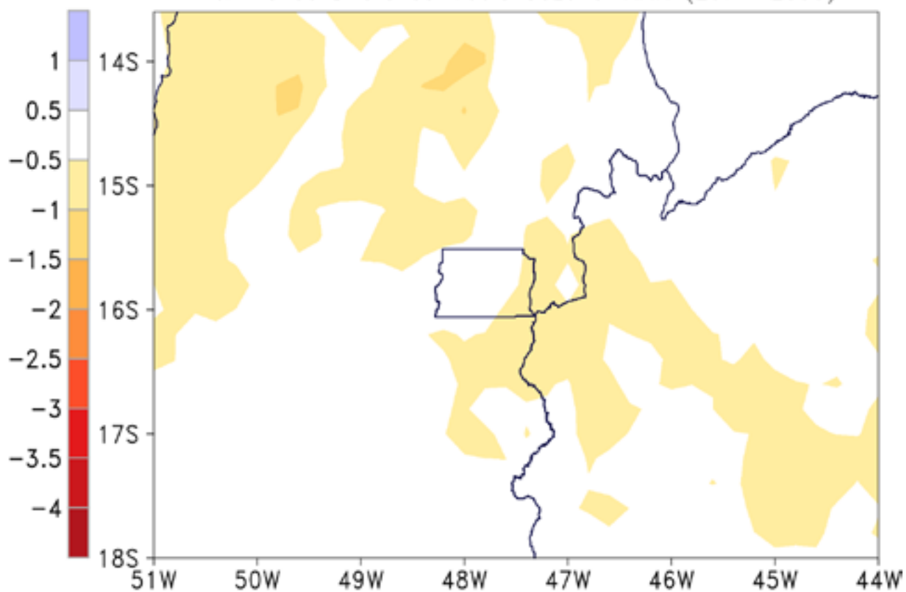
Precipitacao (mm/dia) Eta HadGEM2-ES+MIROC5 20km Maximo da Diferenca Media Sazonal MAM (2071-2099)
