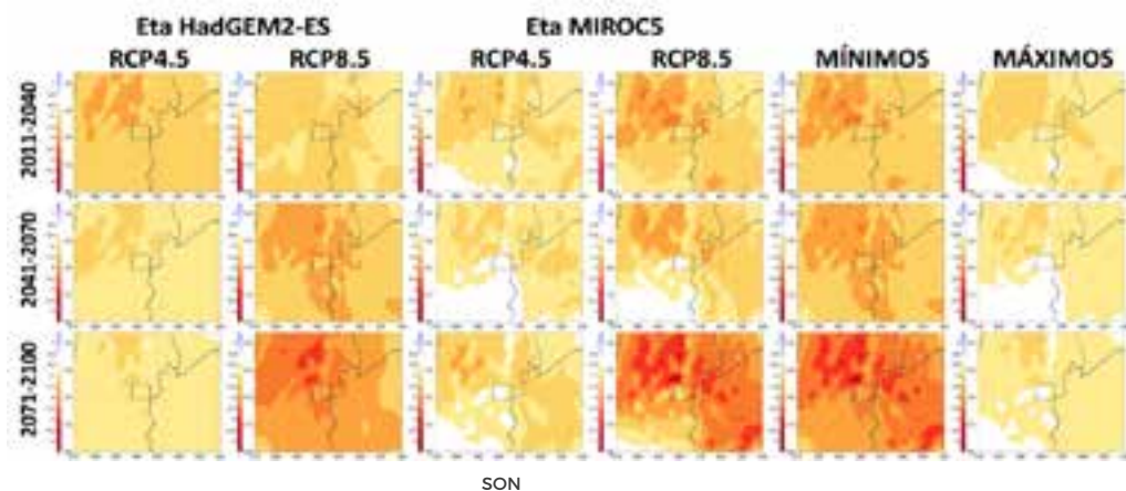
SON
