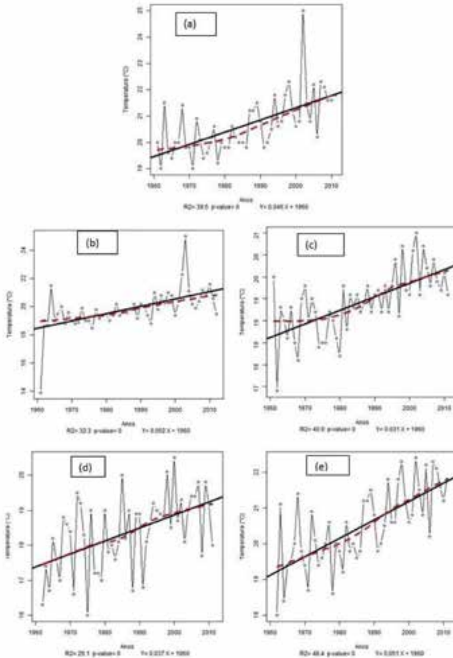
Figura 16 - Índice da Máxima Temperatura Mínima (TminX): (a) anual; (b) verão; (c) outono, (d) inverno e (e) primavera.
